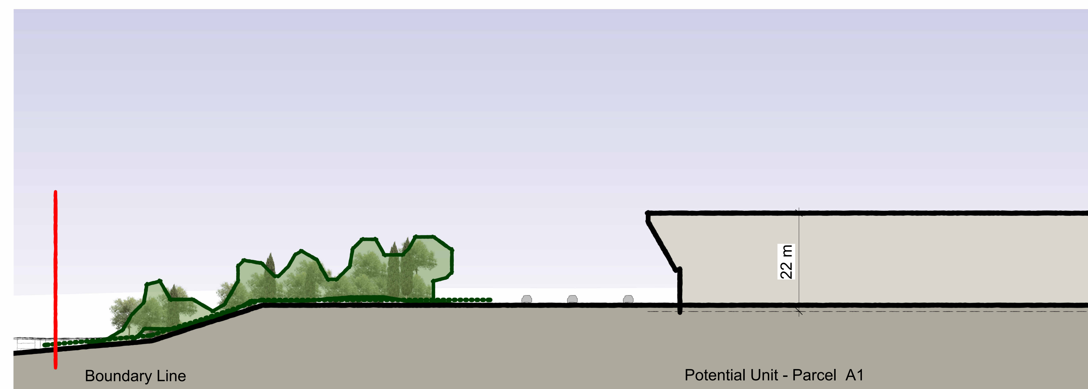
Section C-continuation 2 1 : 500
